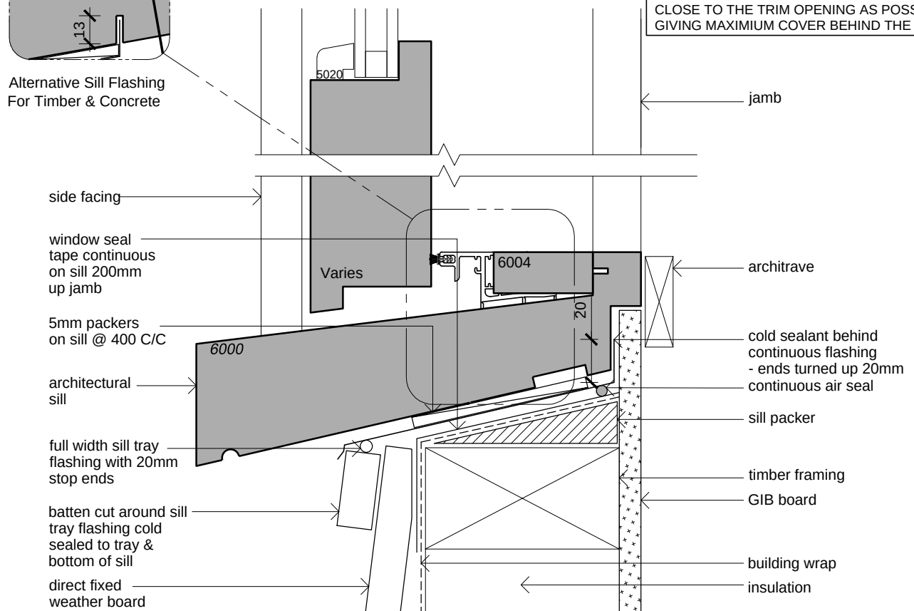
Window Sill Scale: 1:2.5
