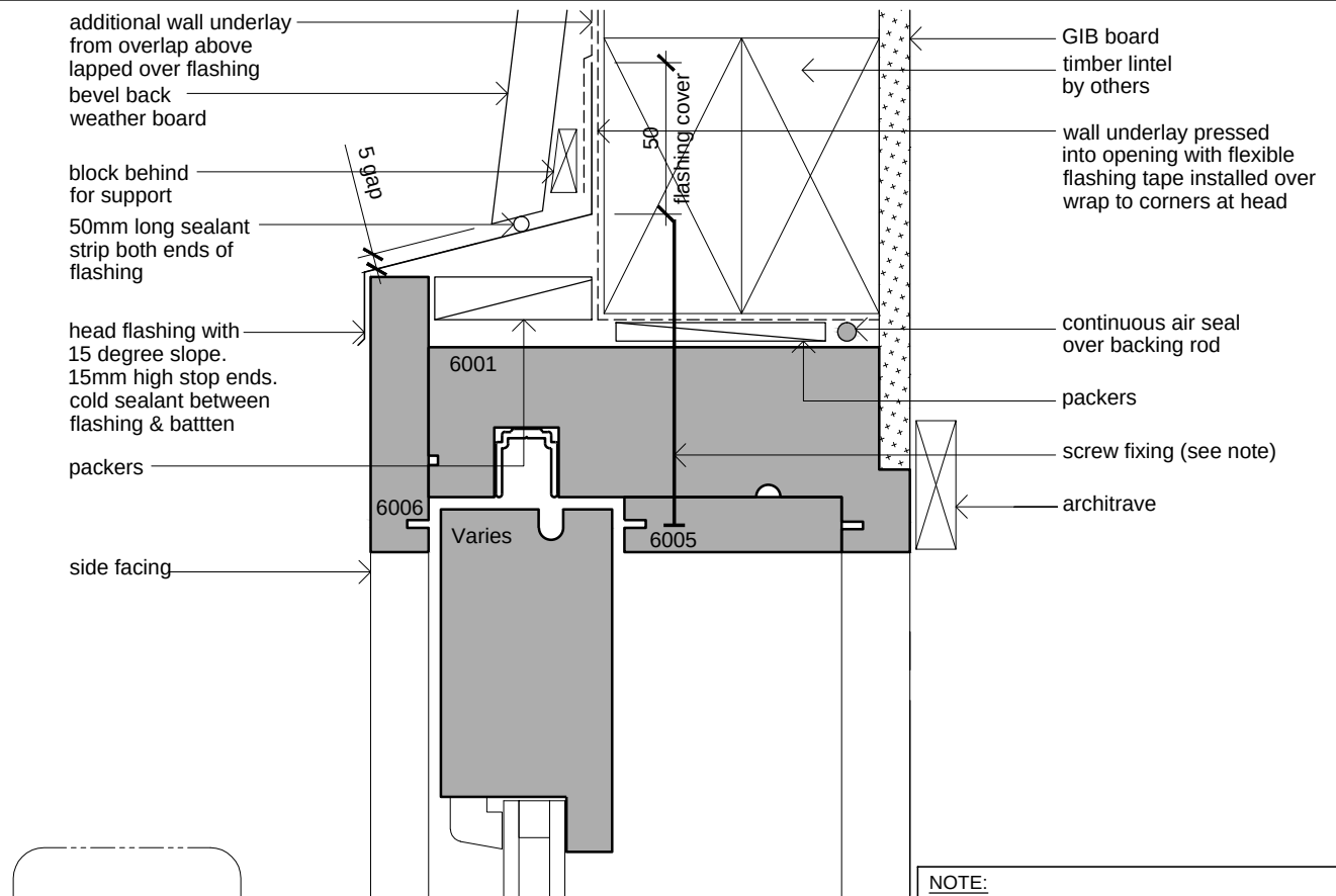
Window Head Scale: 1:2.5
